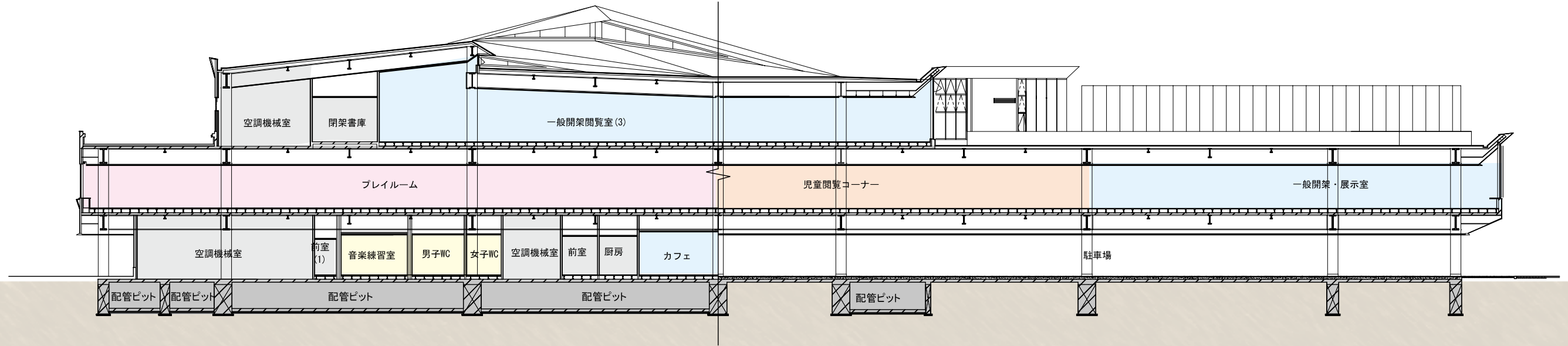
C断面図
