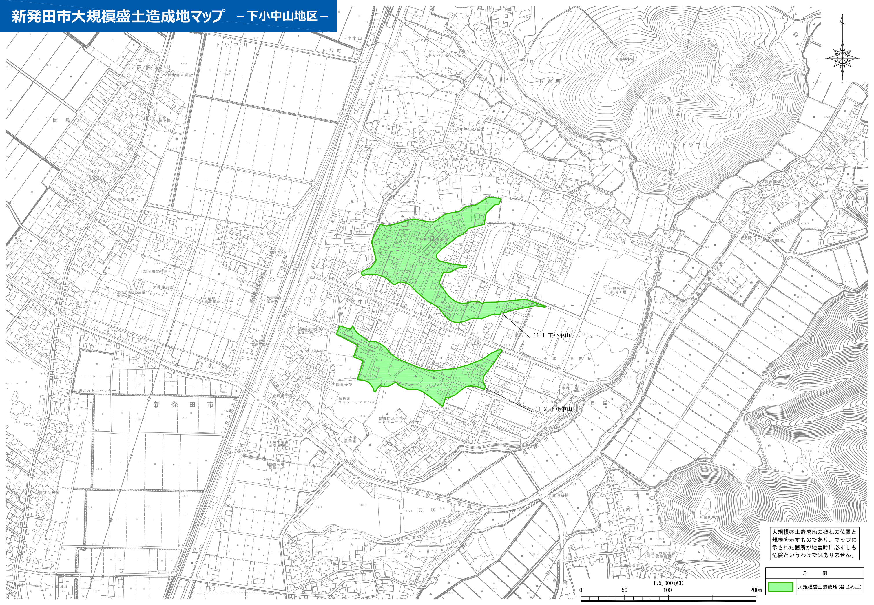
盛土の分類「谷埋め型大規模盛土造成地」
