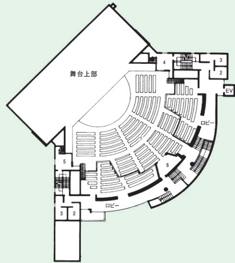
3階平面図
