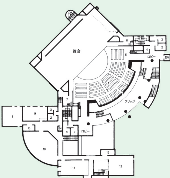
2階平面図
