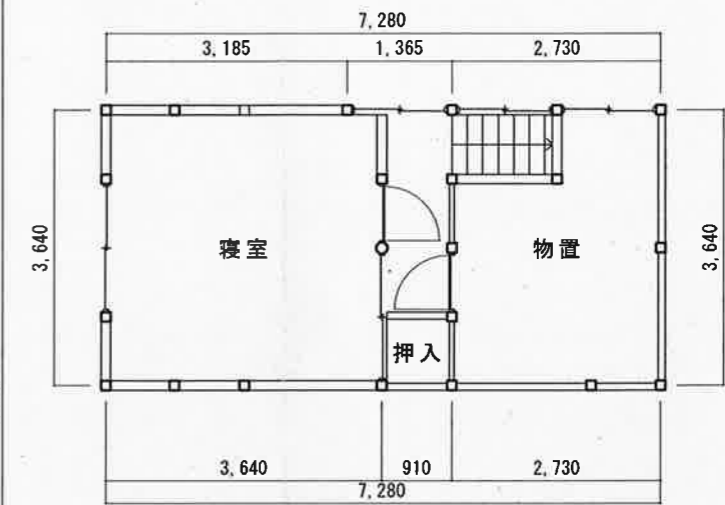
2階平面図 1/100
