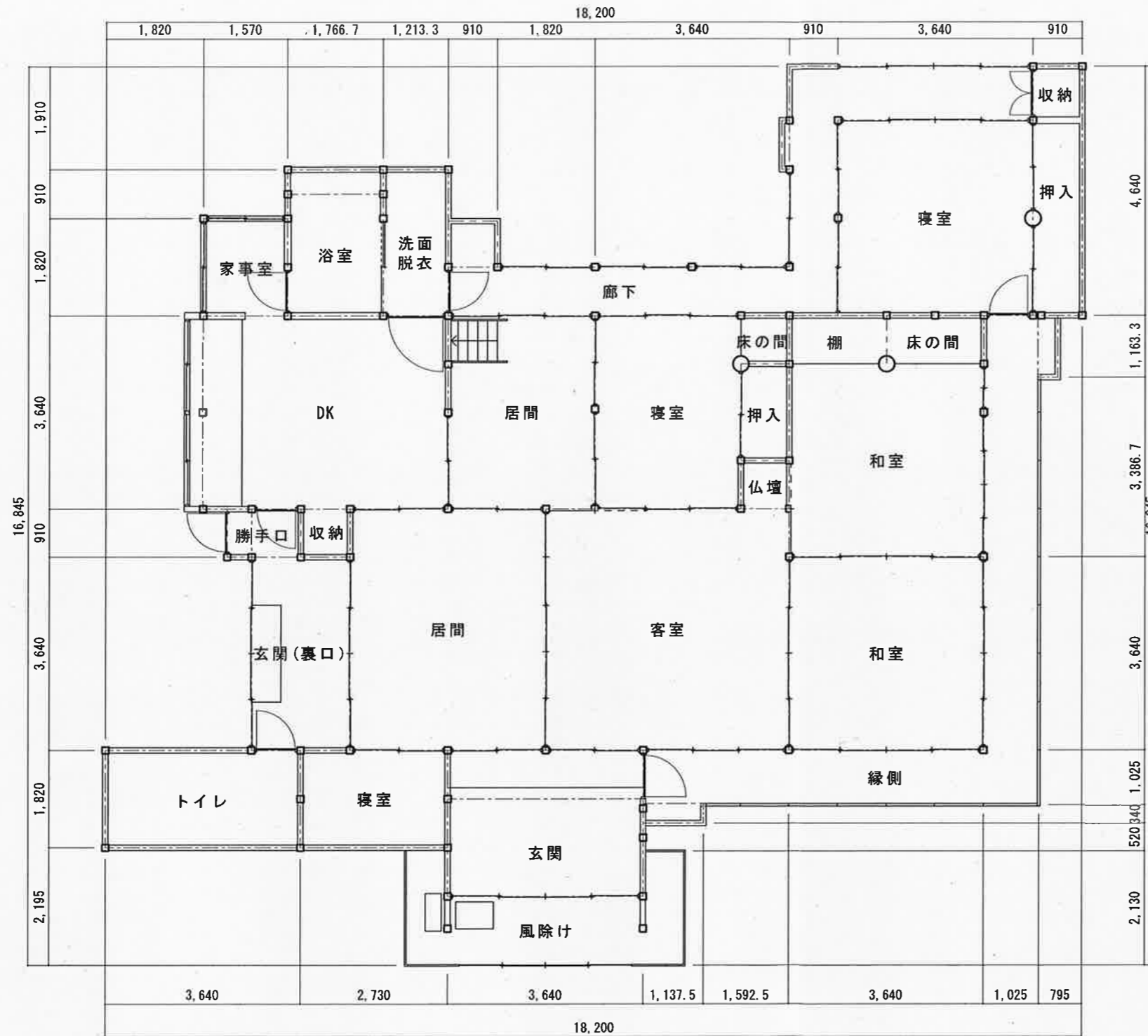
1階平面図 1/100
