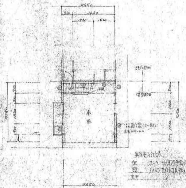
③ 第三層平面圖 S=1/100
