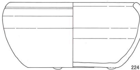
陶磁器実測図見本⑪(土製火鉢)
