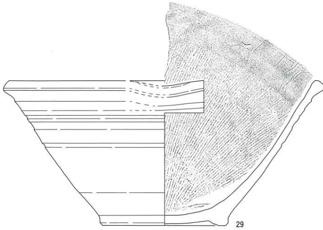
陶磁器実測図見本⑩(陶器播鉢)
