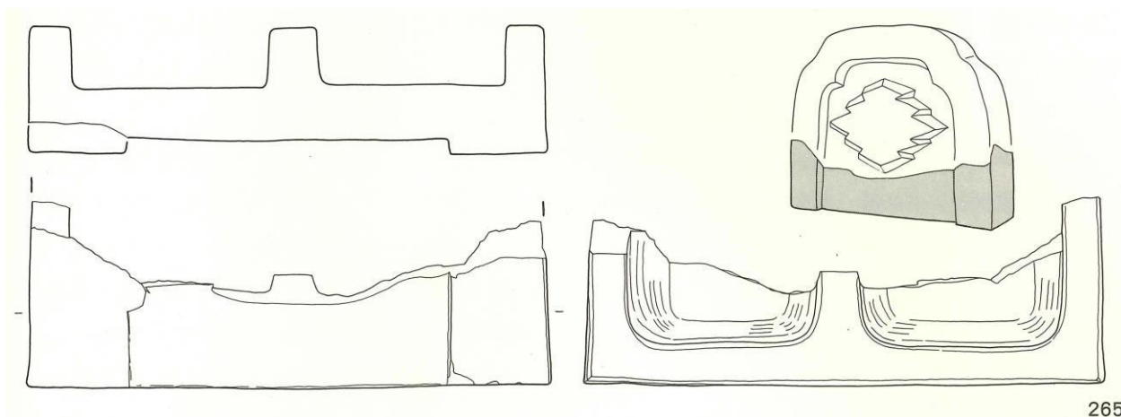
実測図見本③(鬼瓦)
