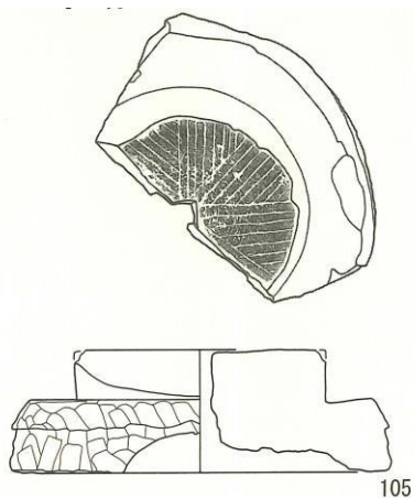
実測図見本③(鬼瓦)
