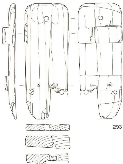
木製品実測図見本⑦(下駄)
