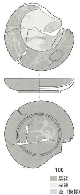
木製品実測図見本⑧(漆器皿)
