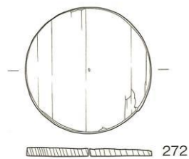
木製品実測図見本④ (曲物底板)
