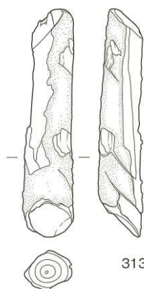
木製品実測図見本⑤ (杭(小))
