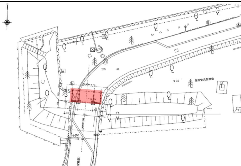
土橋門本体の復元位置
