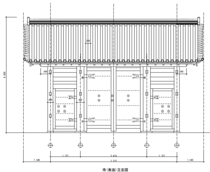
土橋門本体の復元図
