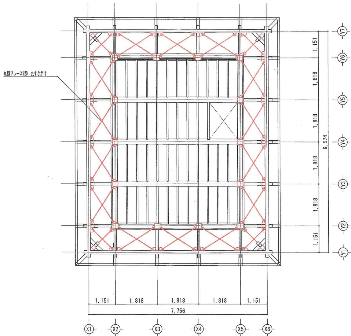
図 3.26 旧二の丸隅櫓 補強案④ 二階床水平ブレース配置図 (S=1/100)
